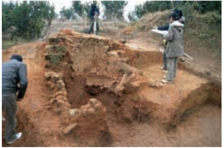
漢代製鉄炉？ (沙子堂遺跡・四川省) Furnace for iron smelting, Han period?(Shazitang,Sichuan)
