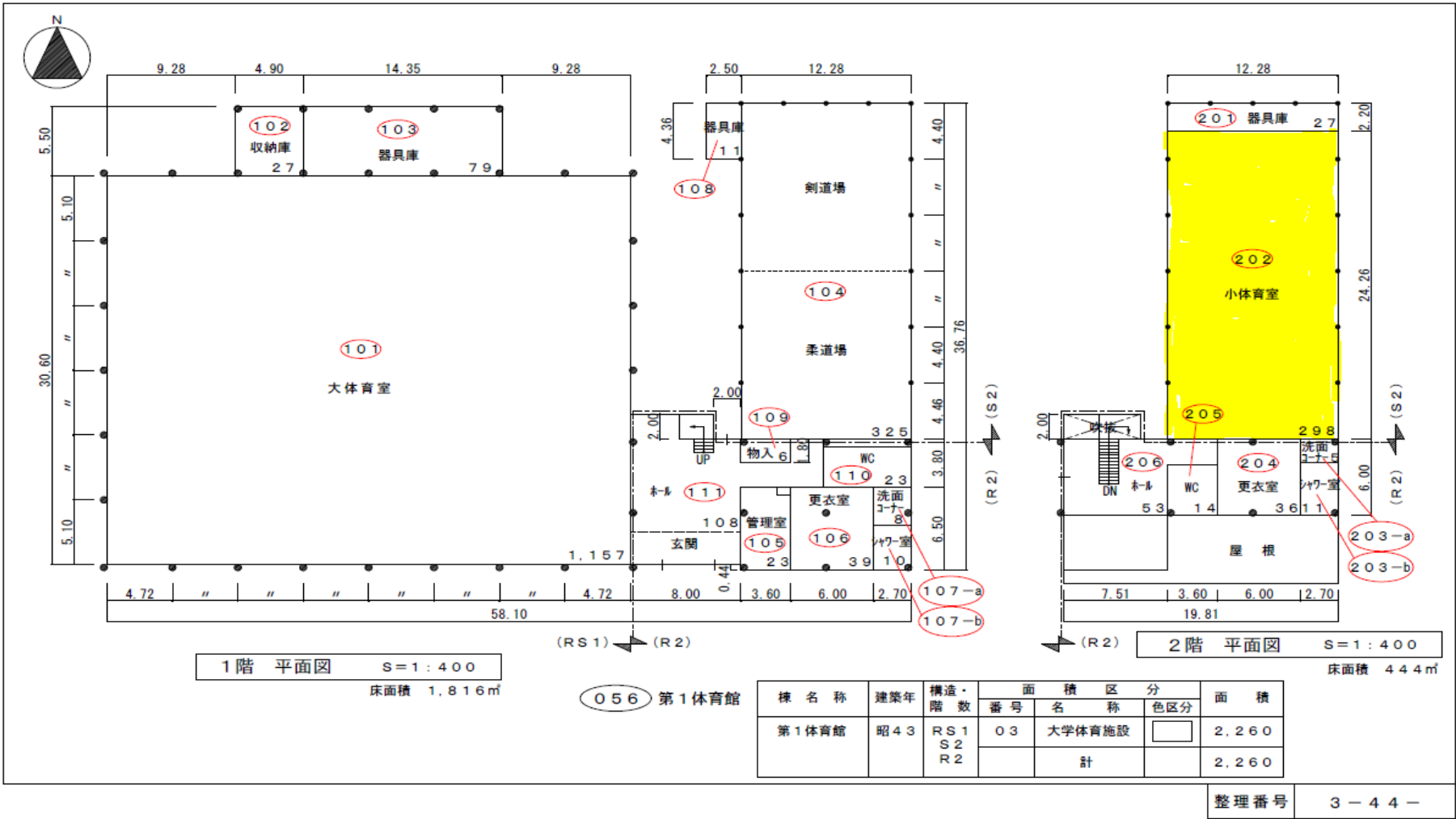
棟 別 平 面 図
