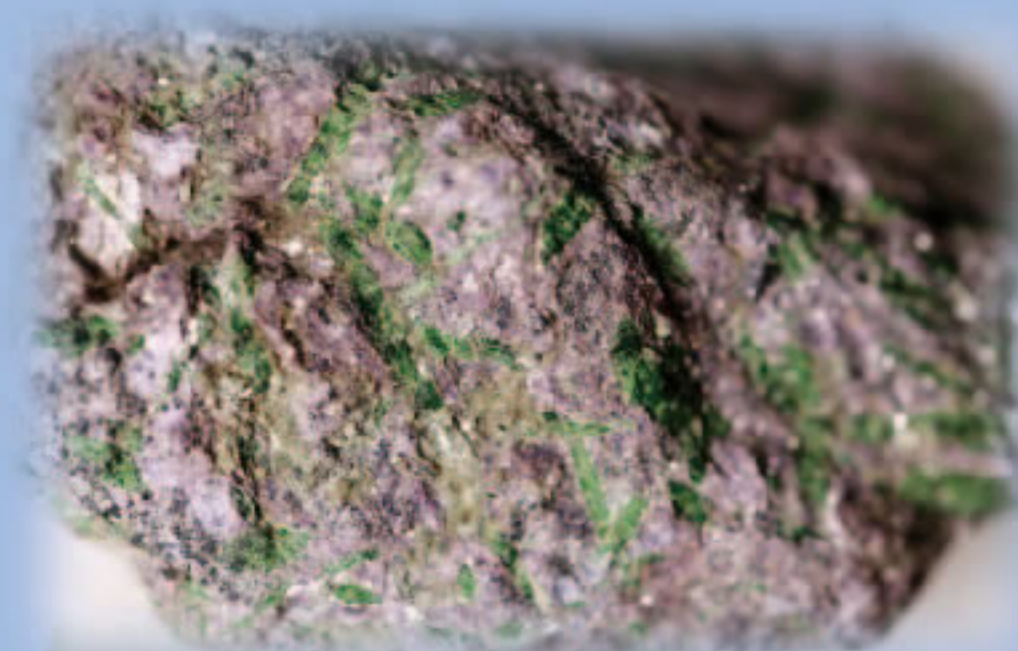
愛媛閃石
