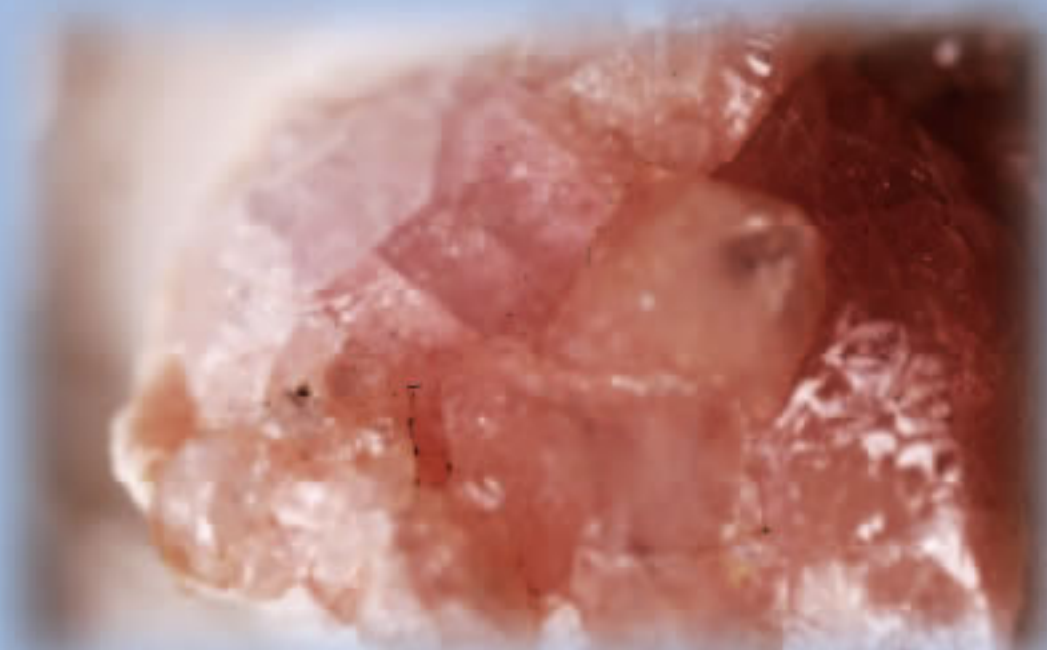
魚眼石
