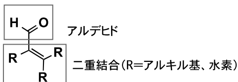
不飽和アルデヒド
