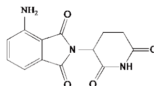
図9. ポマリドミドの化学構造
