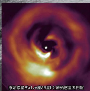
原始惑星ぎょしゃ座AB星bと原始惑星系円盤
