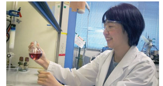
新たに合成された赤色色素
