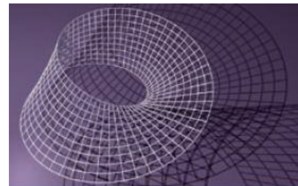
メビウスの帯
