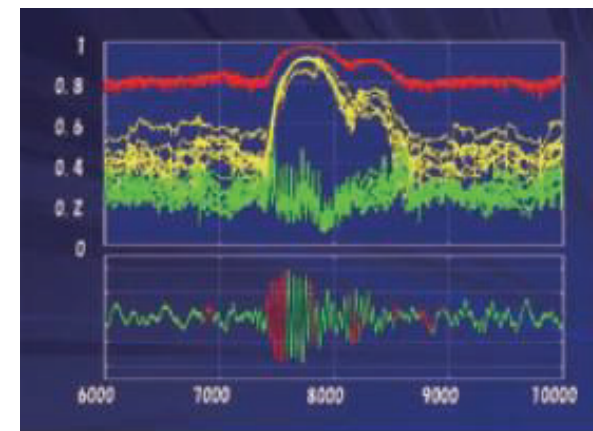
数理的に解析された地震波
