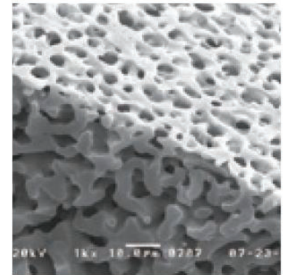
多孔体の電子顕微鏡写真
