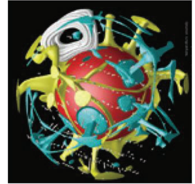
地球の内部の 流体力学シミュレーション
